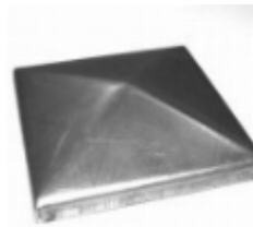
Заглушка, арт. 15.059 150x150x1мм Вес: 0.25 кг Цена: 140 руб.
