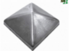
Заглушка на столб 60x60, арт. 15.055.02 60x60x1мм Вес: 0.043 кг Цена: 17 руб.
