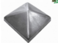
Заглушка на столб 60x60, арт. 15.055.36 60x60x1мм Вес: 0.03 кг Цена: 22 руб.
